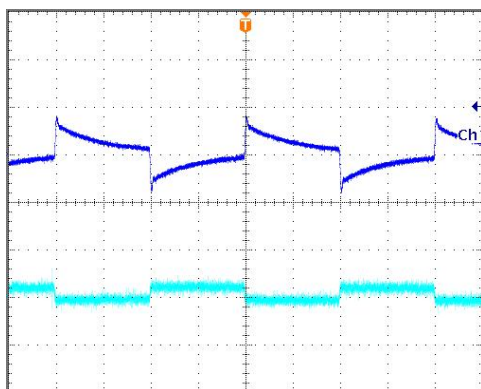
动态响应
