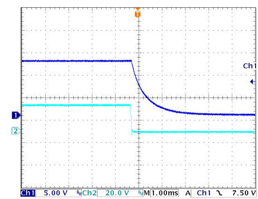
关机特性
