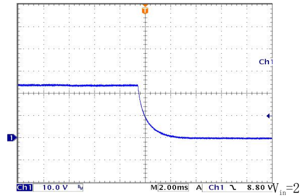
关机特性
