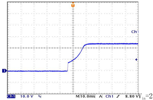
典型启动建立时间
