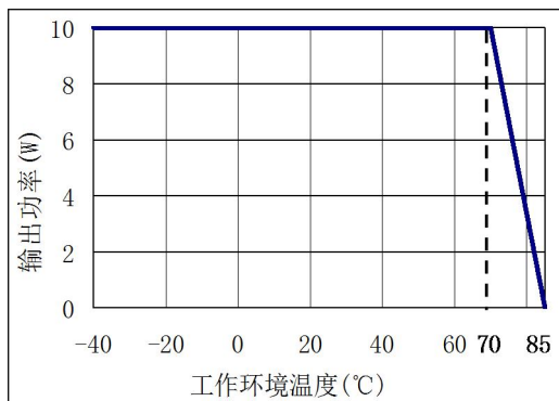
自然冷却降额曲线
