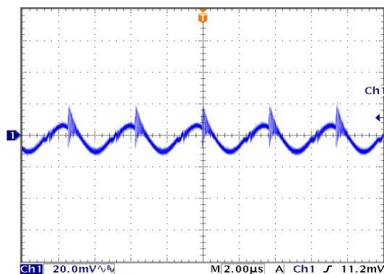
典型输出纹波
