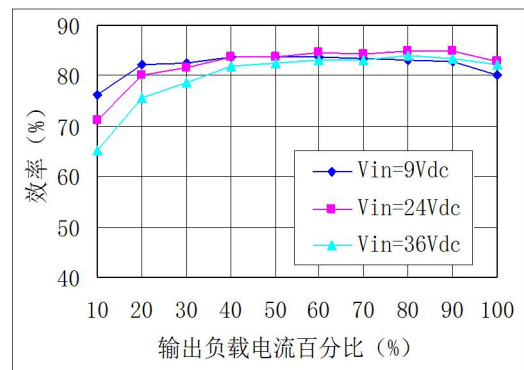
典型效率曲线
