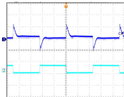
动态响应
