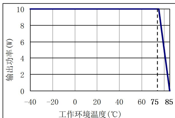
自然冷却降额曲线
