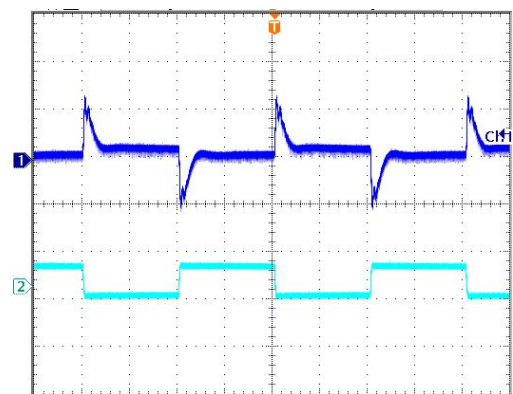
动态响应
