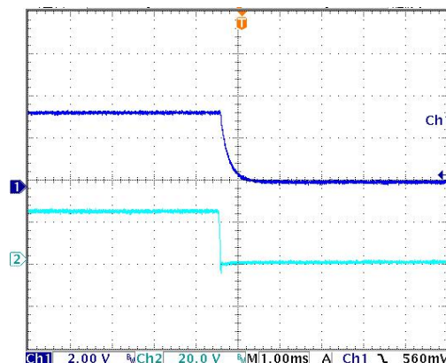
关机特性
