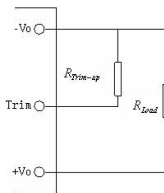
输出电压上调连线图
