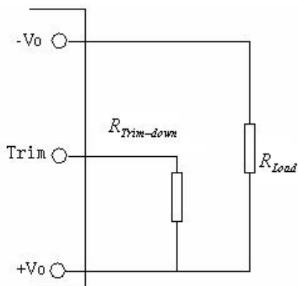
输出电压下调连线图
