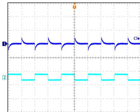
动态响应
