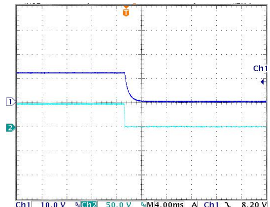
关机特性
