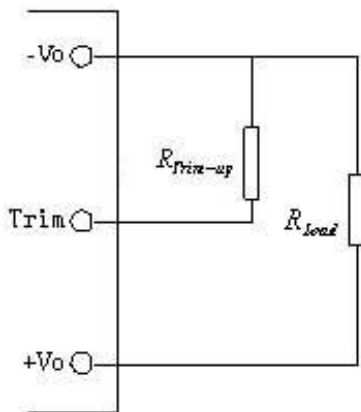
输出电压上调连线图
