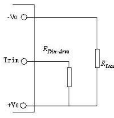
输出电压下调连线图
