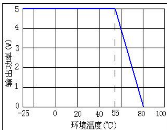
自然冷却降额曲线
