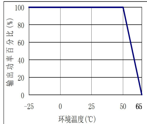
自然冷却降额曲线
