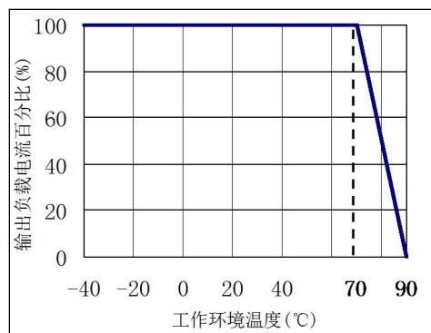
自然冷却降额曲线
