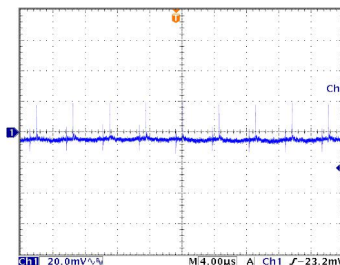
典型输出纹波(V02)
