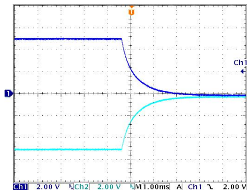
关机特性
