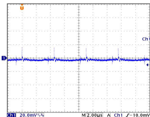
典型输出纹波(V01)
