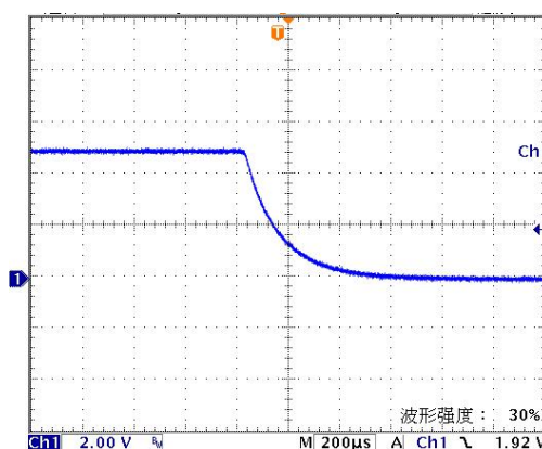
关机特性
