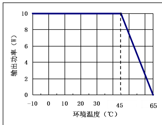
降额曲线
