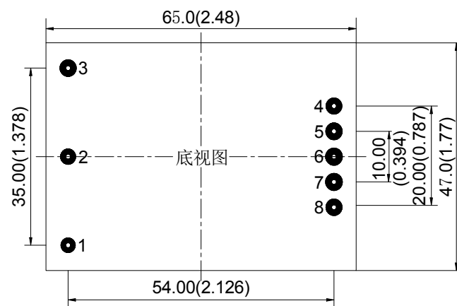
印制板布板推荐
