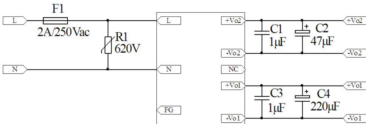
基本应用连线
