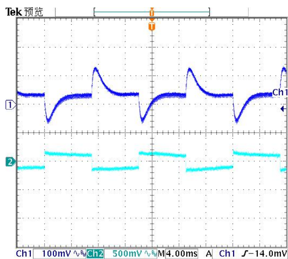
典型输出波纹
