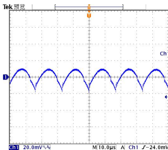
典型输出波纹
