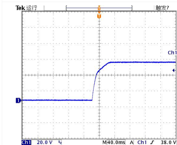
典型输出建立时间
